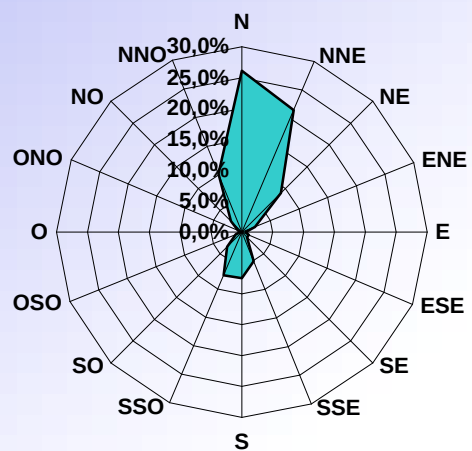
DISTRIBUTION ORIENTATION DU VENT AVRIL 2014
