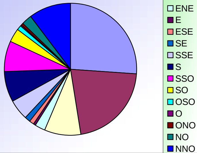
ORIENTATIONS DES VENTS AVRIL 2014
