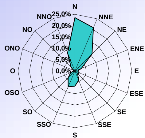
DISTRIBUTION ORIENTATION DU VENT JUILLET 2014
