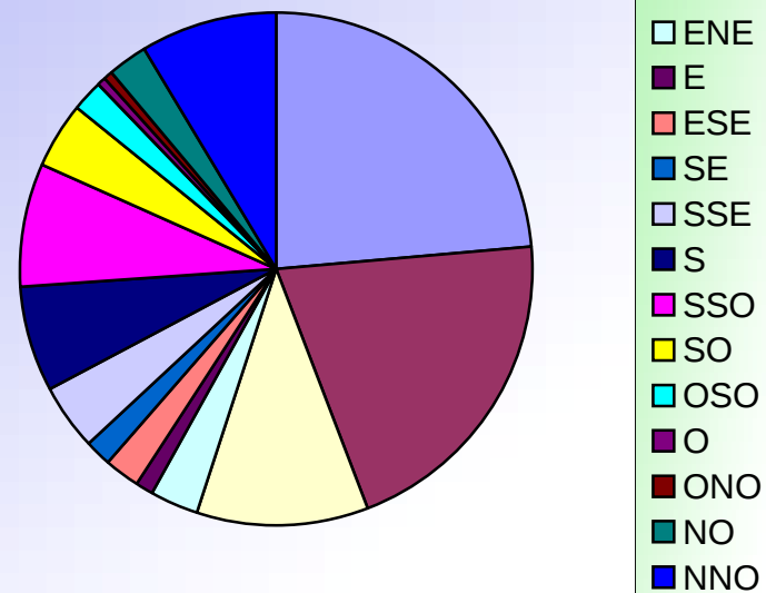
ORIENTATIONS DES VENTS JUILLET 2014
