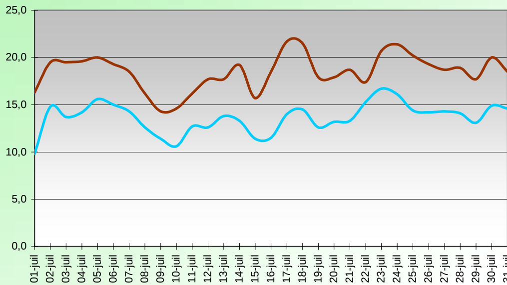
RAFALE MAXI (Km/H) JUILLET 2014
