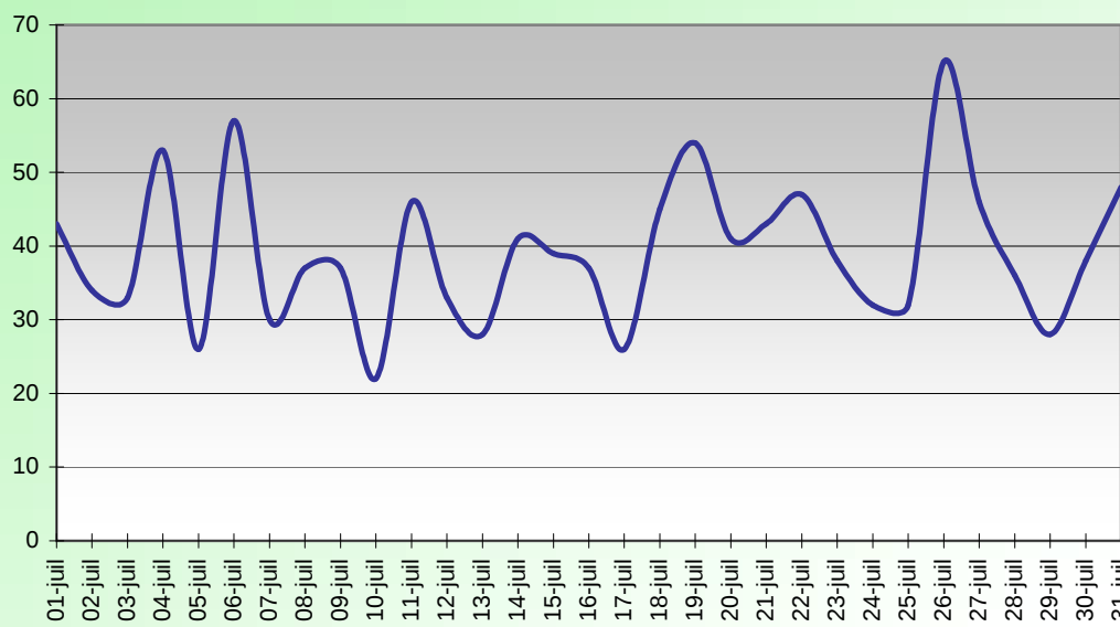
RAFALE MAXI (Km/H) JUILLET 2014
