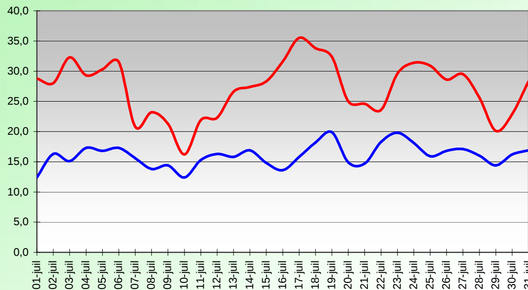
HUMIDITE RELATIVE (%) JUILLET 2014
