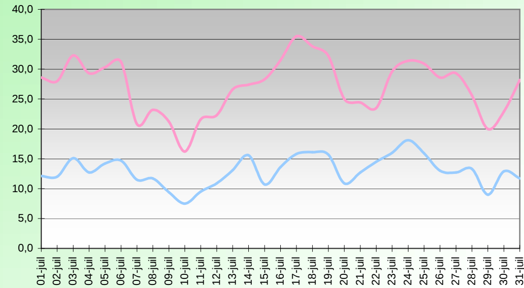
WINDCHILL (°C) JUILLET 2014
