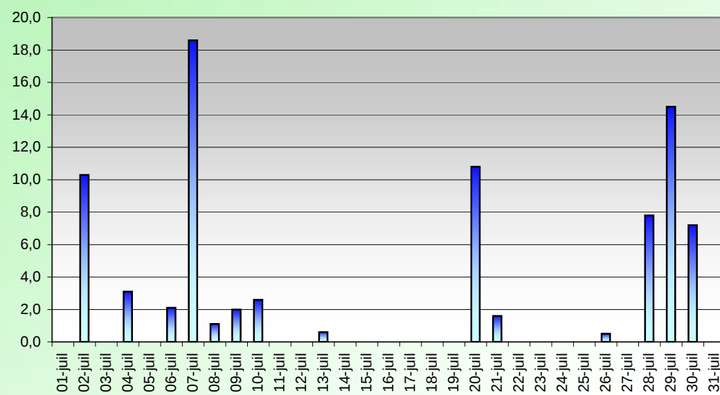
PRECIPITATIONS (mm) JUILLET 2014
