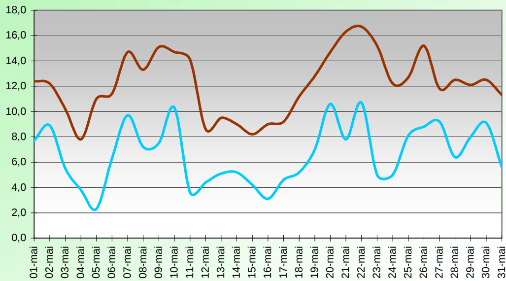
RAFALE MAXI (Km/H) MAI 2014
