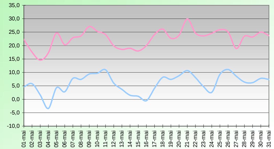
WINDCHILL (°C) MAI 2014
