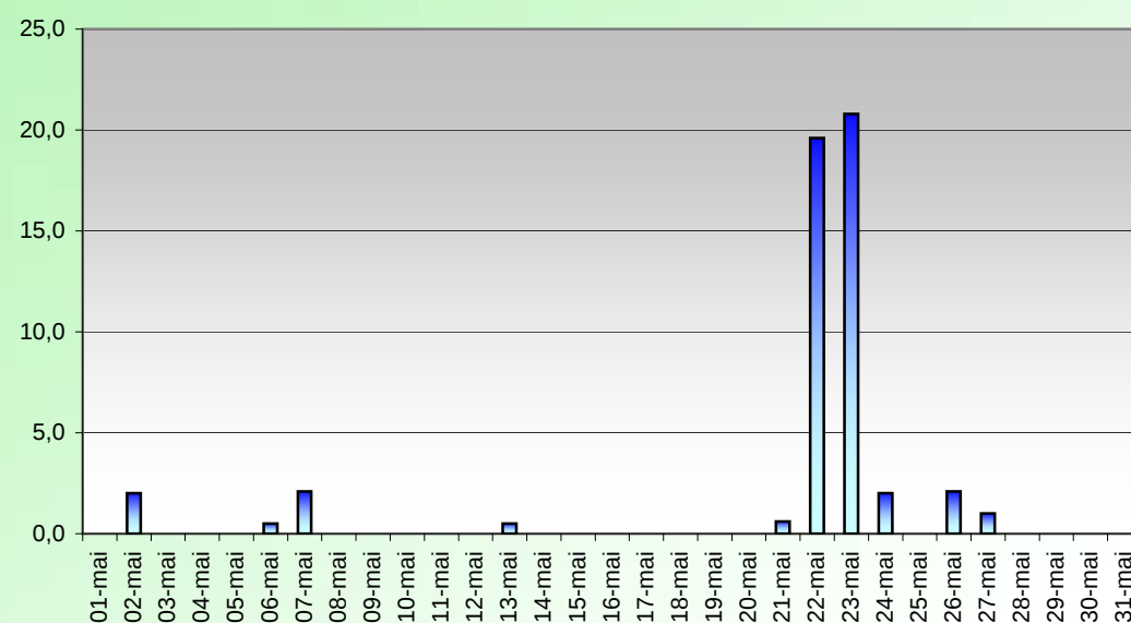
PRECIPITATIONS (mm) MAI 2014
