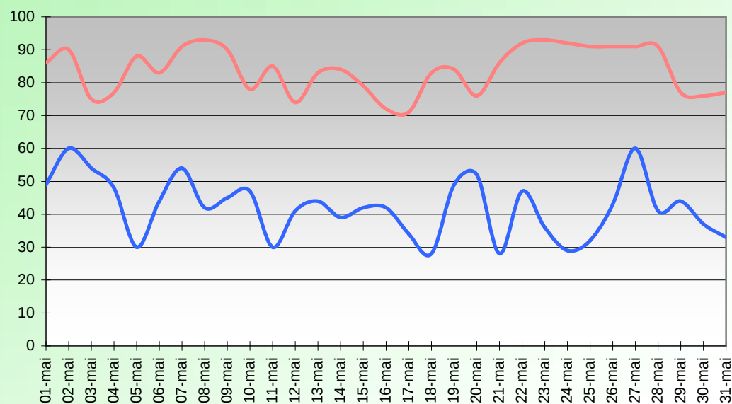
HUMIDITE RELATIVE (%) MAI 2014
