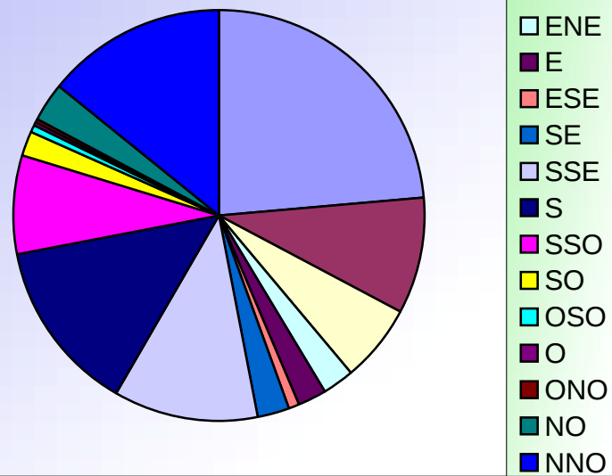
ORIENTATIONS DES VENTS AVRIL 2015
