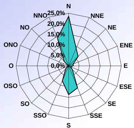
DISTRIBUTION ORIENTATION DU VENT AVRIL 2015
