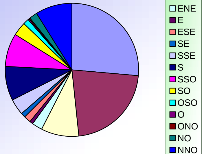
ORIENTATIONS DES VENTS JANVIER 2015
