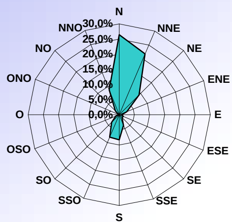
DISTRIBUTION ORIENTATION DU VENT JANVIER 2015
