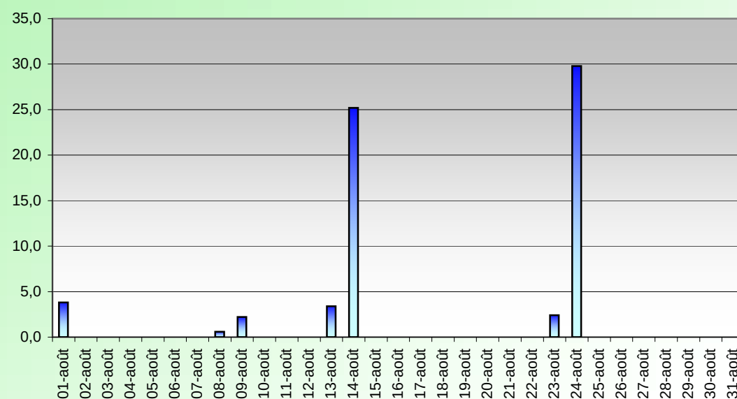
PRECIPITATIONS (mm) AOÛT 2015
