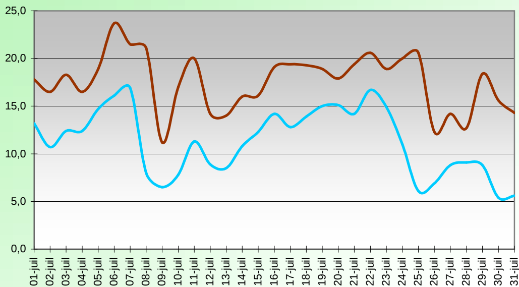
WINDCHILL OU TEMPERATURE RESSENTIE (°C) JUILLET 2015
