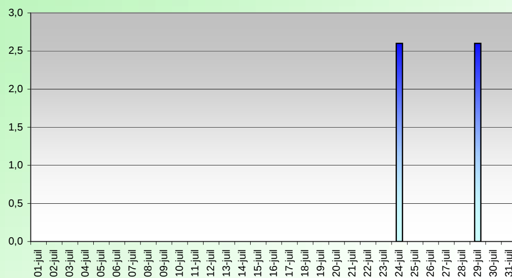
PRECIPITATIONS (mm) JUILLET 2015
