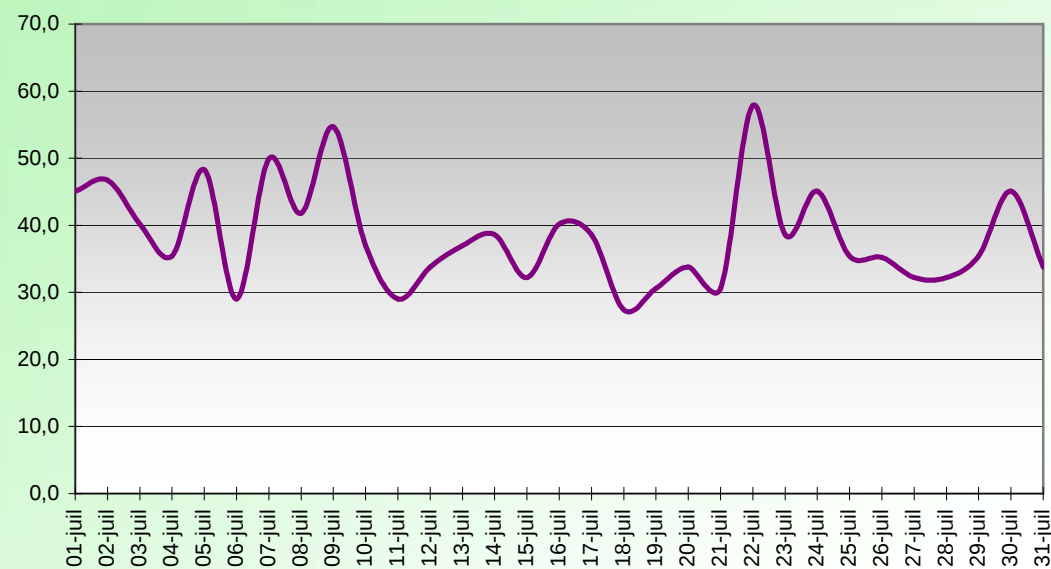
HEAT INDEX OU INDICE DE CHALEUR (°C) JUILLET 2015
