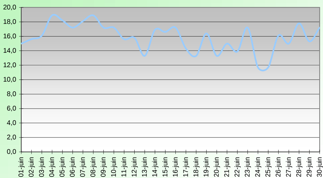
WINDCHILL OU TEMPERATURE RESSENTIE (°C) JUIN 2015
