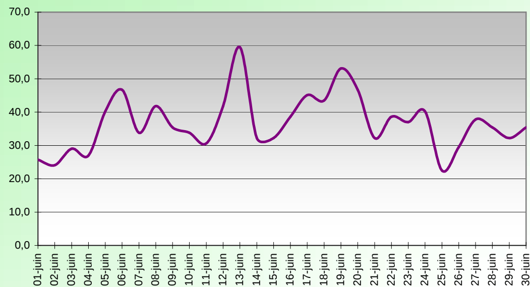
HEAT INDEX OU INDICE DE CHALEUR (°C) JUIN 2015
