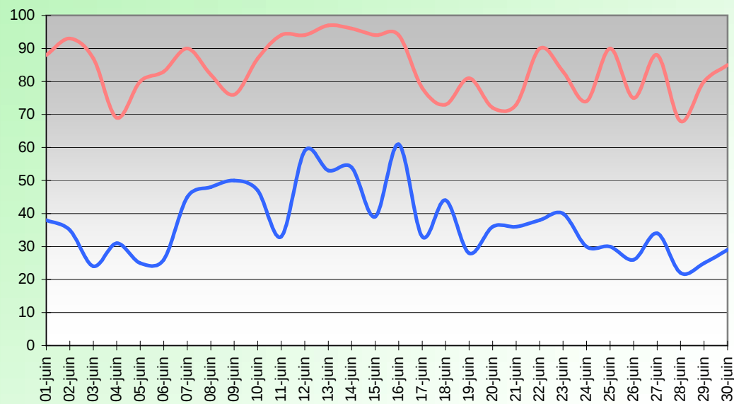
HUMIDITE RELATIVE (%) JUIN 2015
