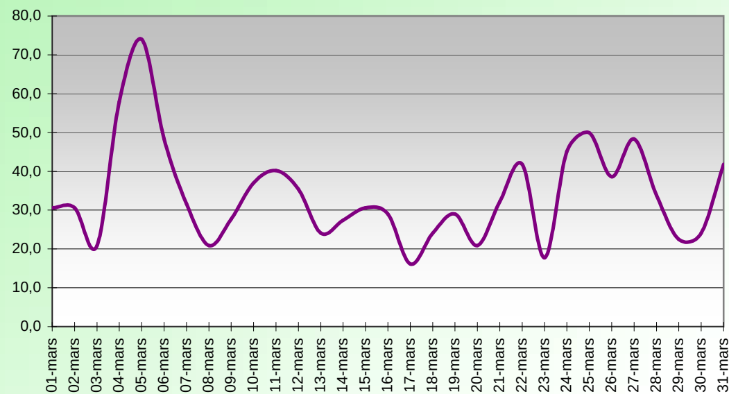
HEAT INDEX OU INDICE DE CHALEUR (°C) MARS 2015
