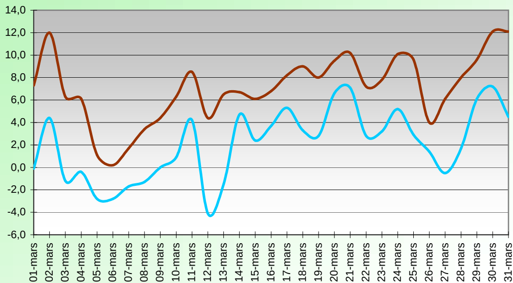
WINDCHILL OU TEMPERATURE RESSENTIE (°C) MARS 2015
