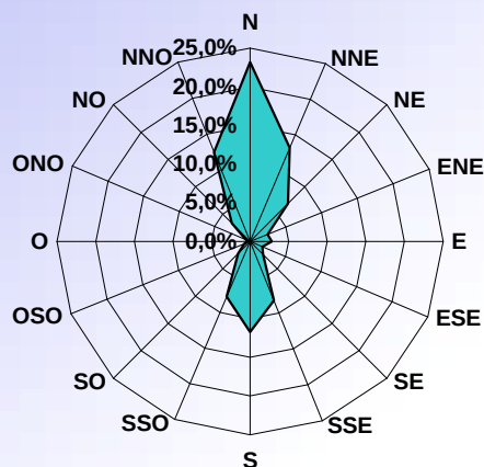
DISTRIBUTION ORIENTATION DU VENT ANNEE 2016
