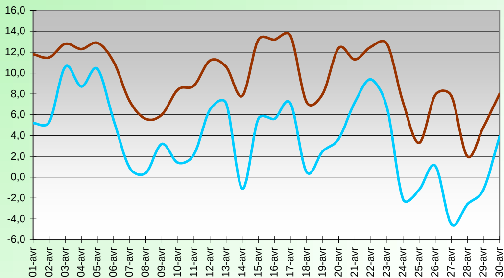
WINDCHILL OU TEMPERATURE RESSENTIE (°C) AVRIL 2016
