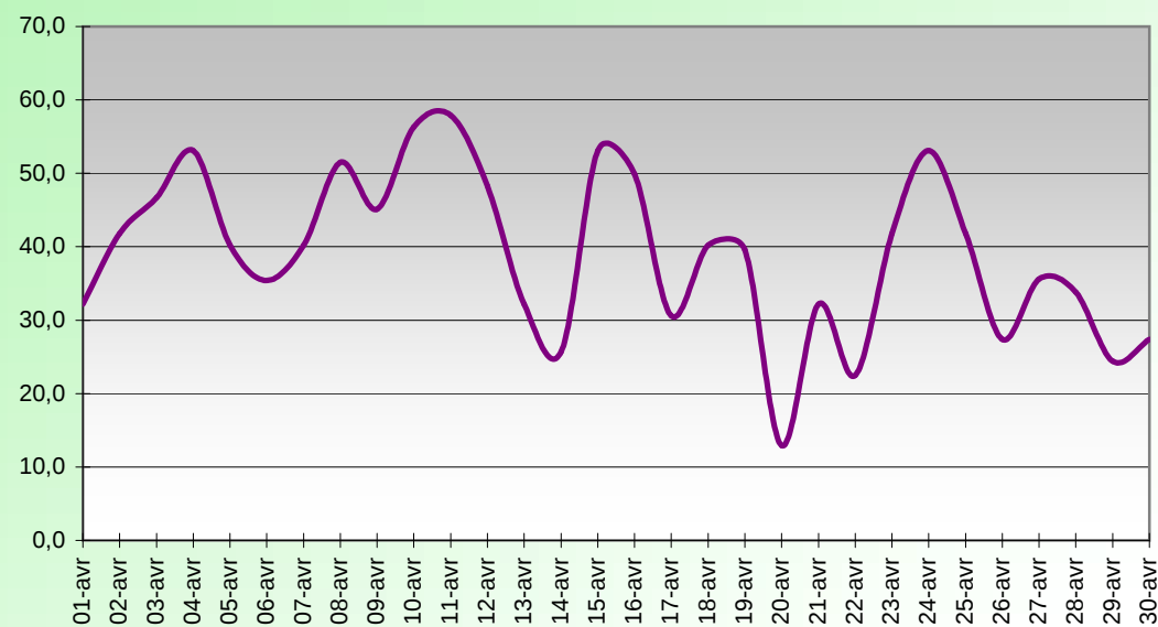
HEAT INDEX OU INDICE DE CHALEUR (°C) AVRIL 2016
