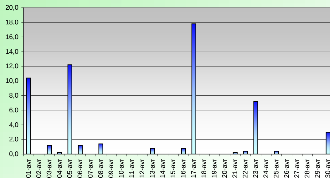
PRECIPITATIONS (mm) AVRIL 2016
