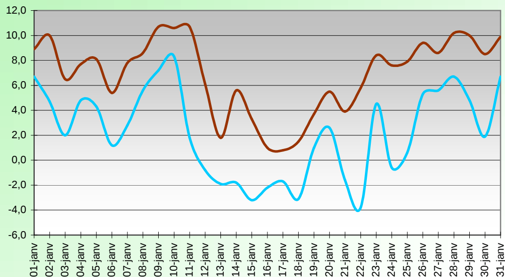
WINDCHILL OU TEMPERATURE RESSENTIE (°C) JANVIER 2016
