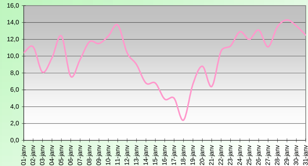
HEAT INDEX OU INDICE DE CHALEUR (°C) JANVIER 2016
