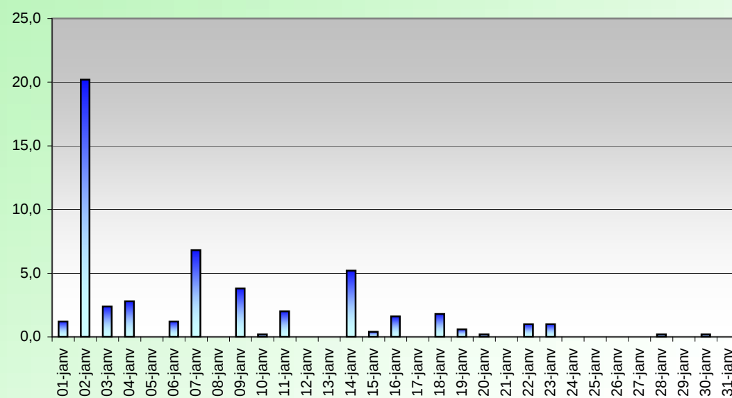
PRECIPITATIONS (mm) JANVIER 2016
