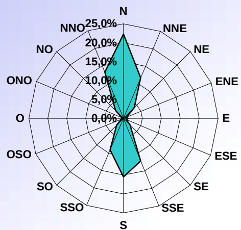
DISTRIBUTION ORIENTATION DU VENT MARS 2017
