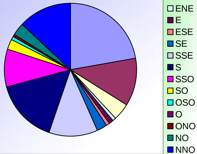
ORIENTATIONS DES VENTS MARS 2017
