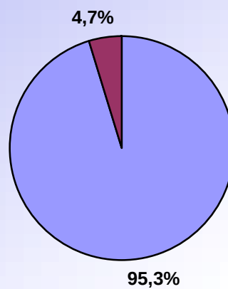
RAPPORT VENT NUL - VENT >0 MARS 2017
