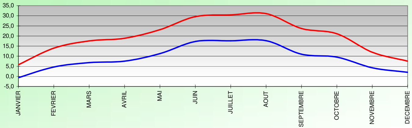
TEMPERATURE (°C) 2017
