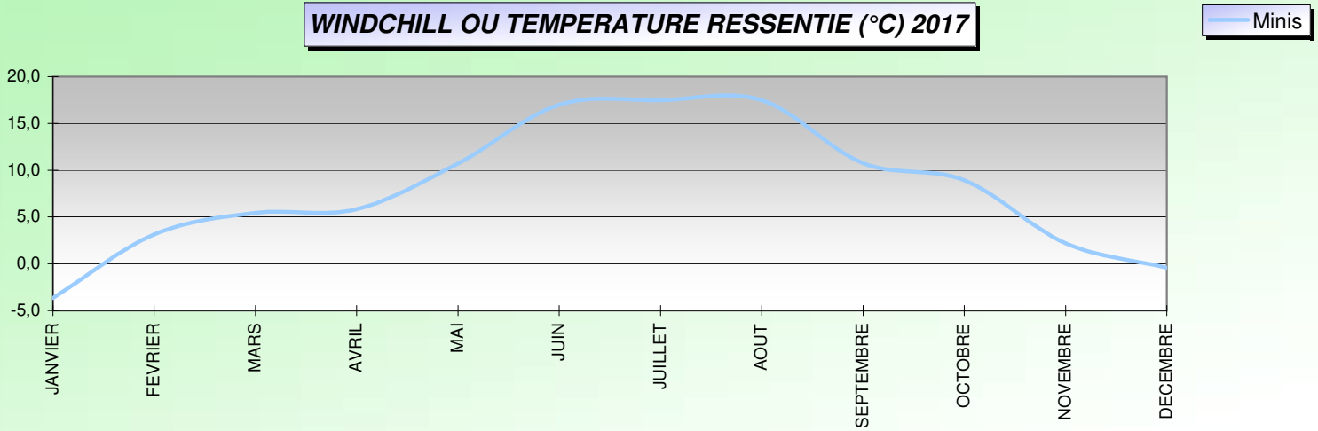
HEAT INDEX OU INDICE DE CHALEUR (°C) 2017
