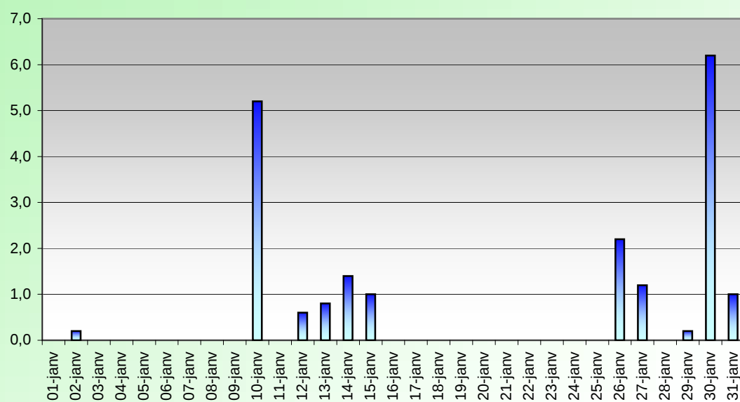
PRECIPITATIONS (mm) JANVIER 2017
