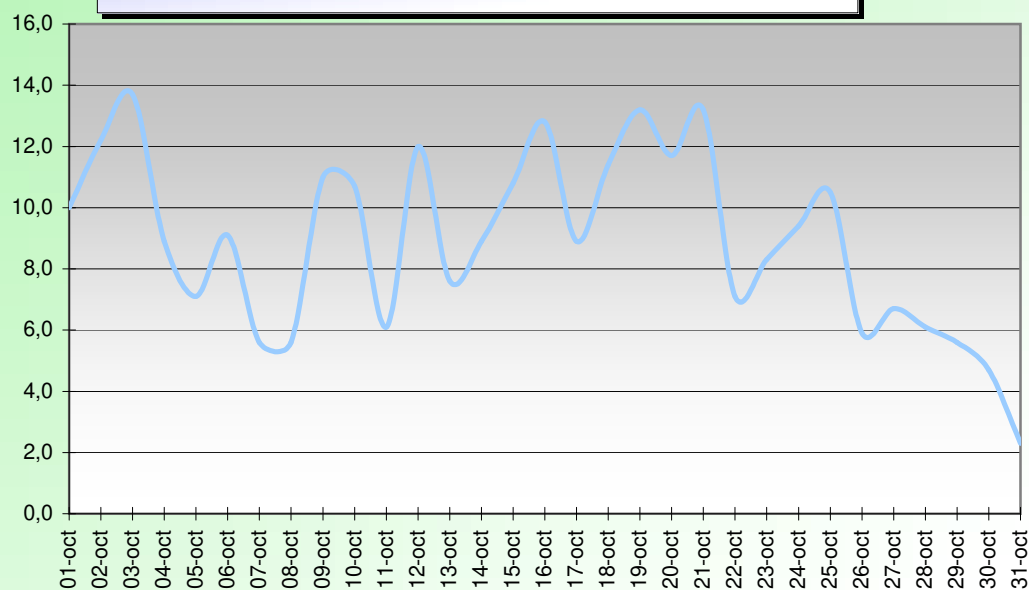
WINDCHILL OU TEMPERATURE RESSENTIE (°C) OCTOBRE 2017
