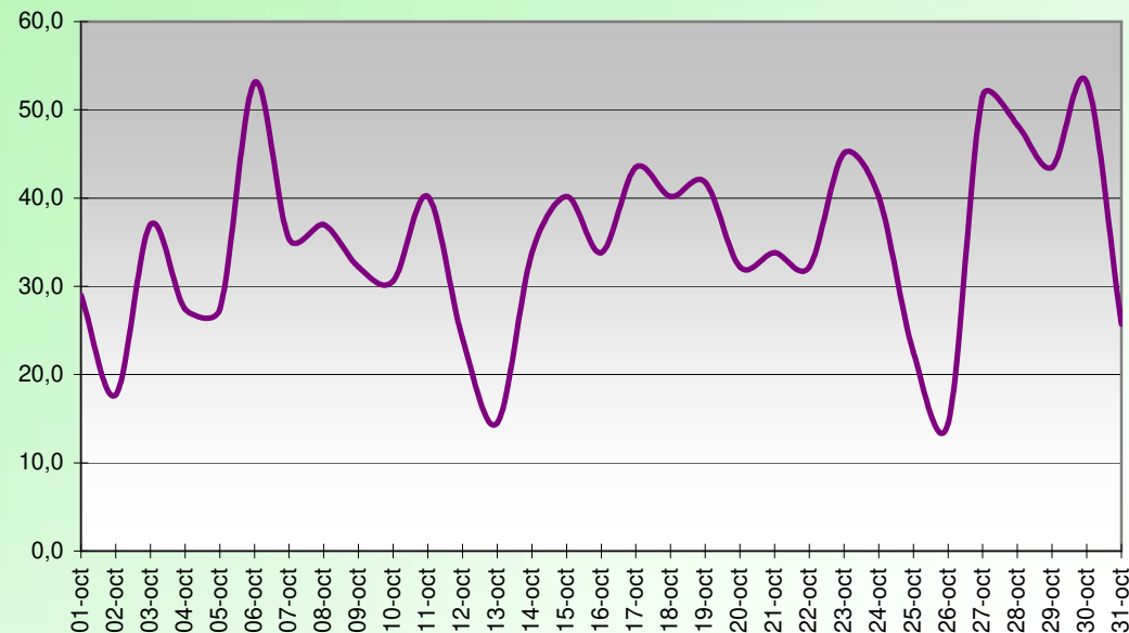
HEAT INDEX OU INDICE DE CHALEUR (°C) OCTOBRE 2017
