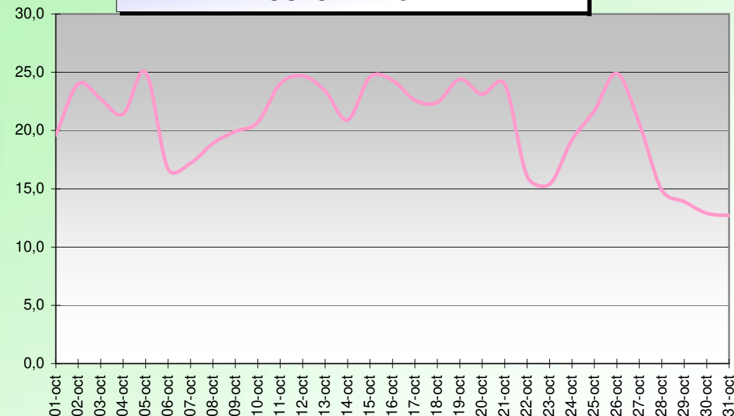
HEAT INDEX OU INDICE DE CHALEUR (°C) OCTOBRE 2017
