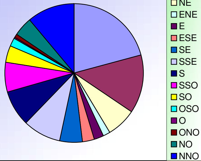
ORIENTATIONS DES VENTS MAI 2018
