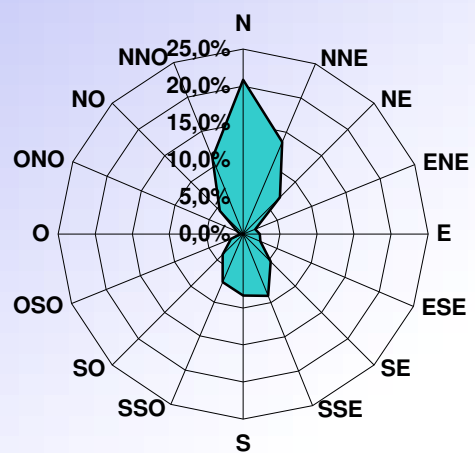
DISTRIBUTION ORIENTATION DU VENT MAI 2018
