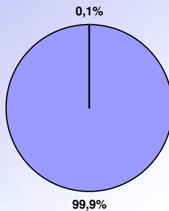
RAPPORT VENT NUL - VENT >0 MAI 2018
