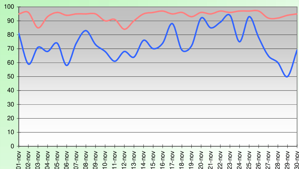
HUMIDITE RELATIVE (%) NOVEMBRE 2018
