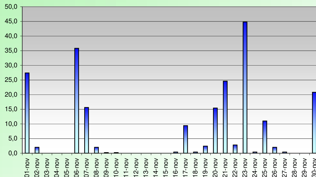
PRECIPITATIONS (mm) NOVEMBRE 2018
