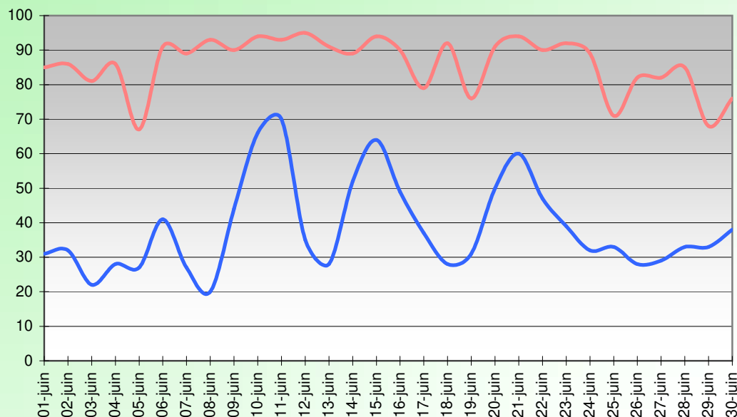
HUMIDITE RELATIVE (%) JUIN 2019
