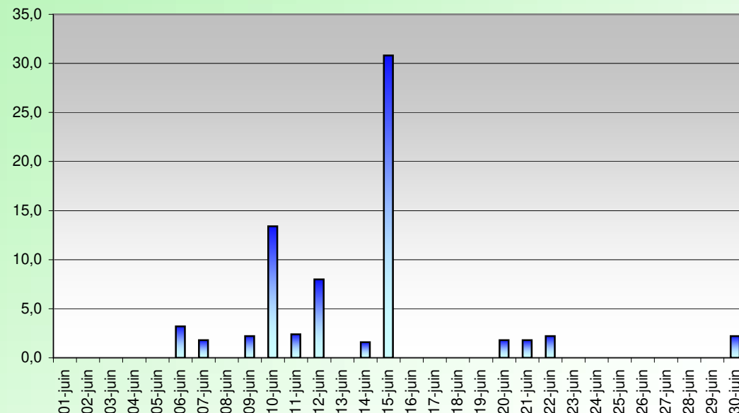
PRECIPITATIONS (mm) JUIN 2019
