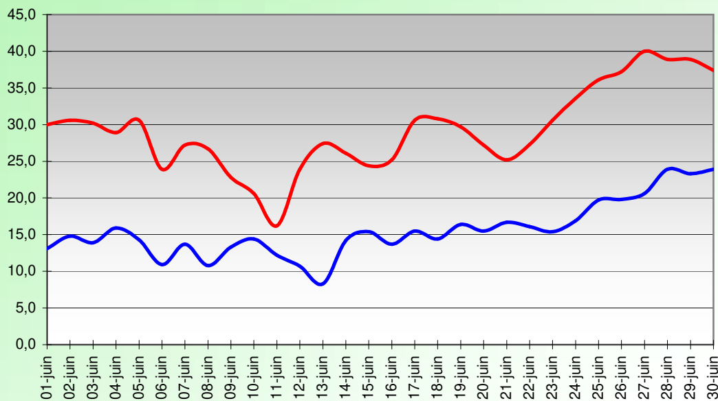
HUMIDITE RELATIVE (%) JUIN 2019
