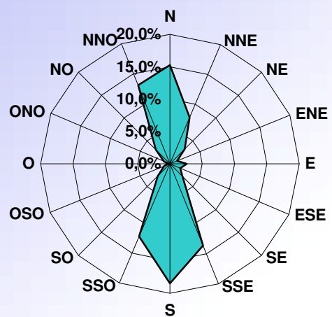
DISTRIBUTION ORIENTATION DU VENT OCTOBRE 2019
