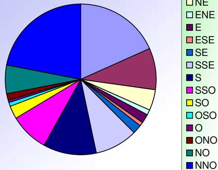
ORIENTATIONS DES VENTS MARS 2020
