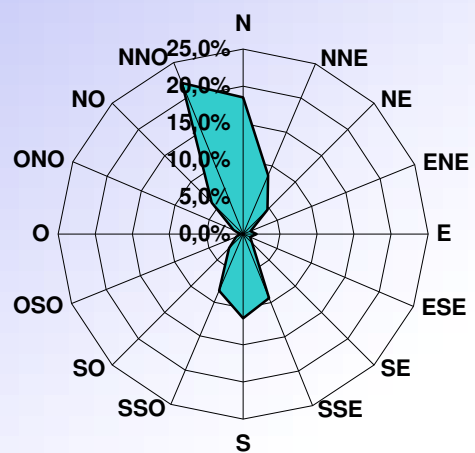
DISTRIBUTION ORIENTATION DU VENT MARS 2020
