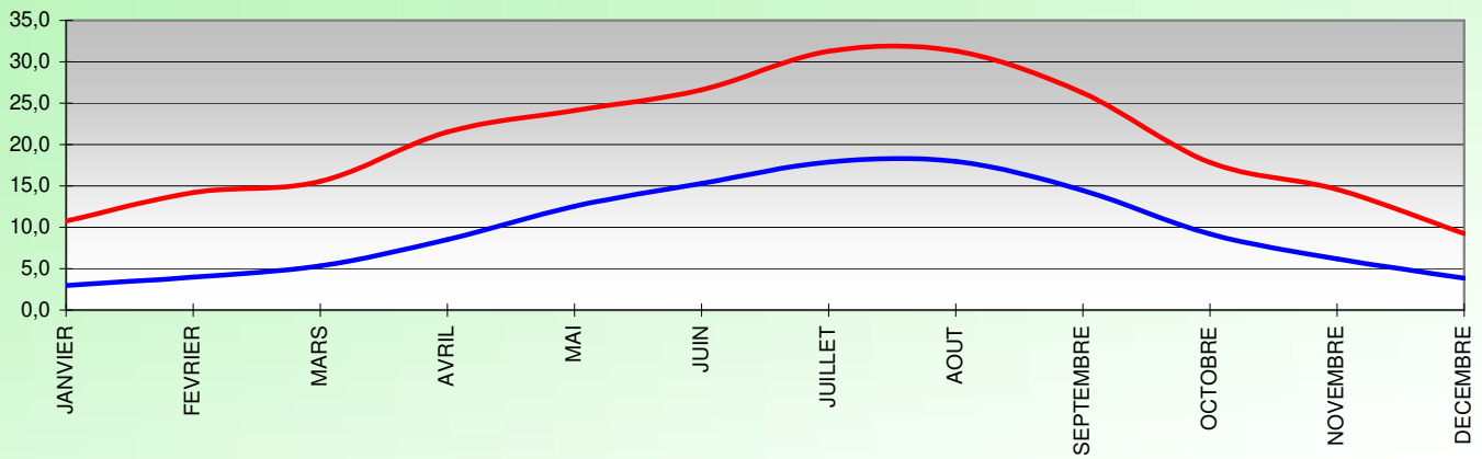
TEMPERATURE (°C) 2020
