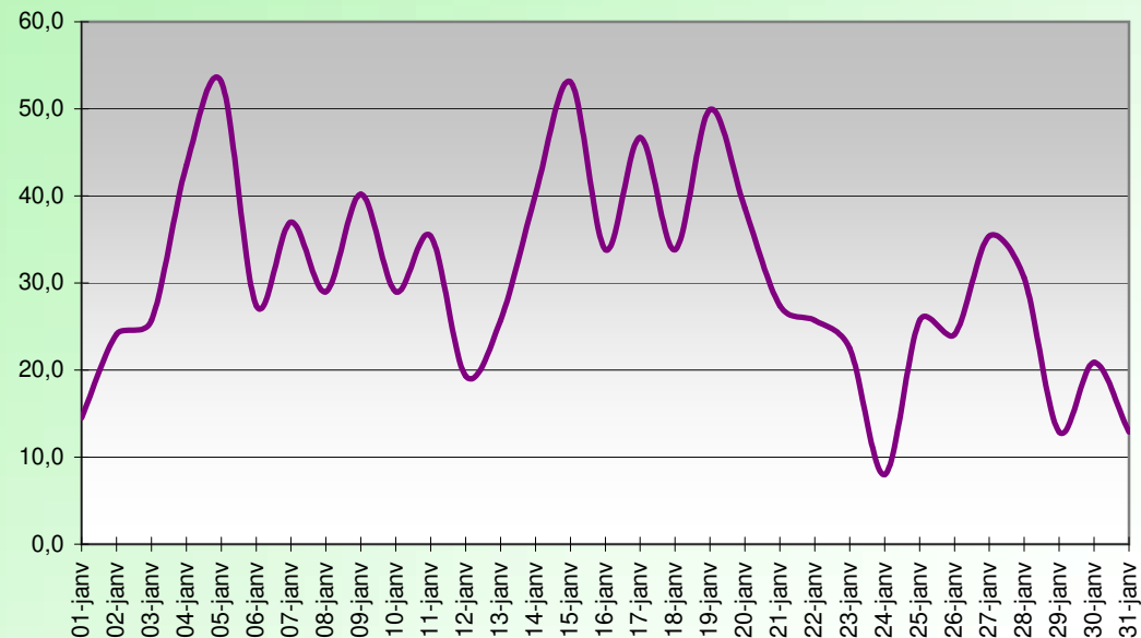
HEAT INDEX OU INDICE DE CHALEUR (°C) JANVIER 2020
