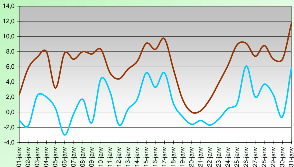
WINDCHILL OU TEMPERATURE RESSENTIE (°C) JANVIER 2020
