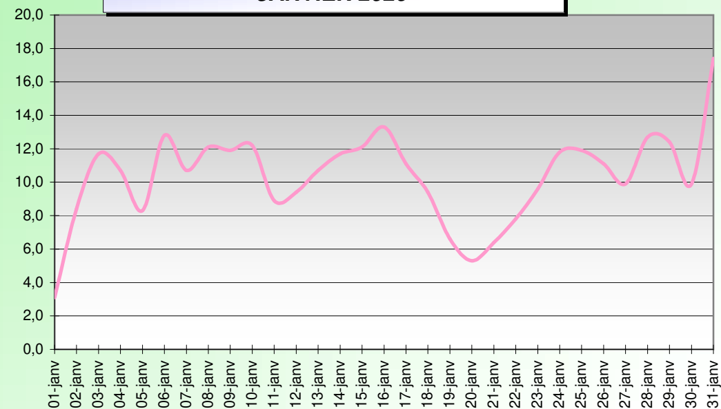
HEAT INDEX OU INDICE DE CHALEUR (°C) JANVIER 2020
