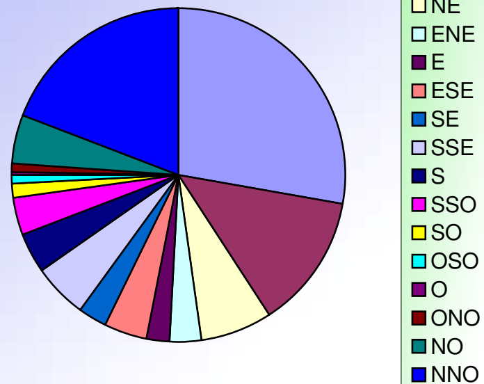
ORIENTATIONS DES VENTS AOUT 2021
