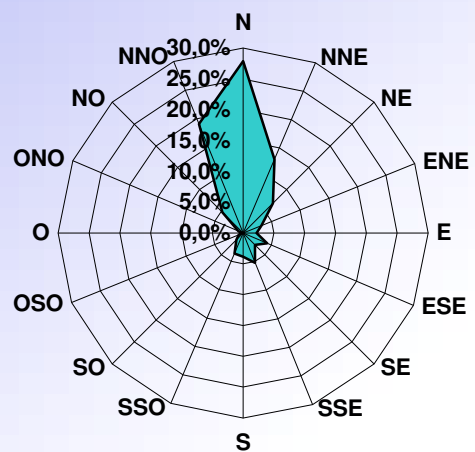
DISTRIBUTION ORIENTATION DU VENT AOUT 2021
