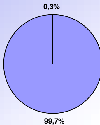
RAPPORT VENT NUL - VENT >0 AOUT 2021
