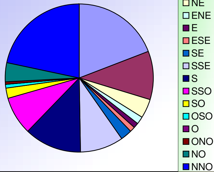
ORIENTATIONS DES VENTS AVRIL 2021
