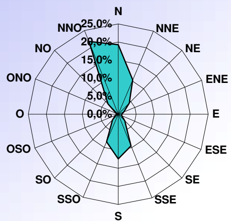
DISTRIBUTION ORIENTATION DU VENT AVRIL 2021
