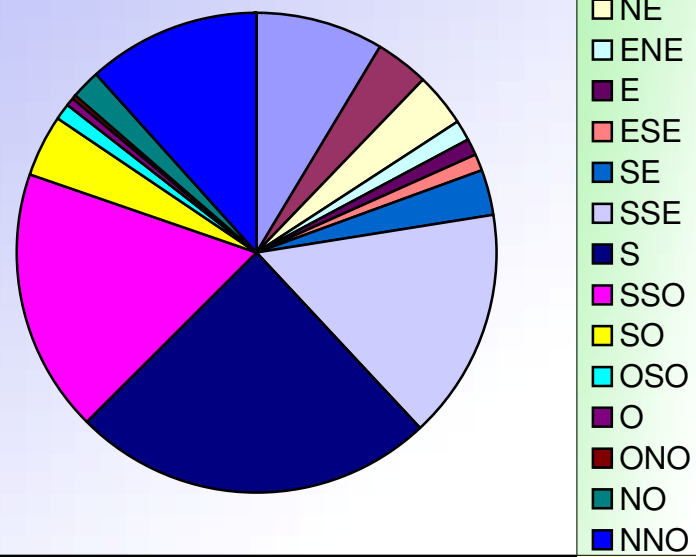
ORIENTATIONS DES VENTS FEVRIER 2021
