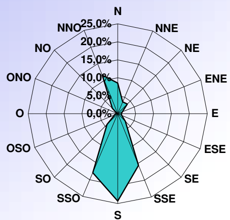
DISTRIBUTION ORIENTATION DU VENT FEVRIER 2021
