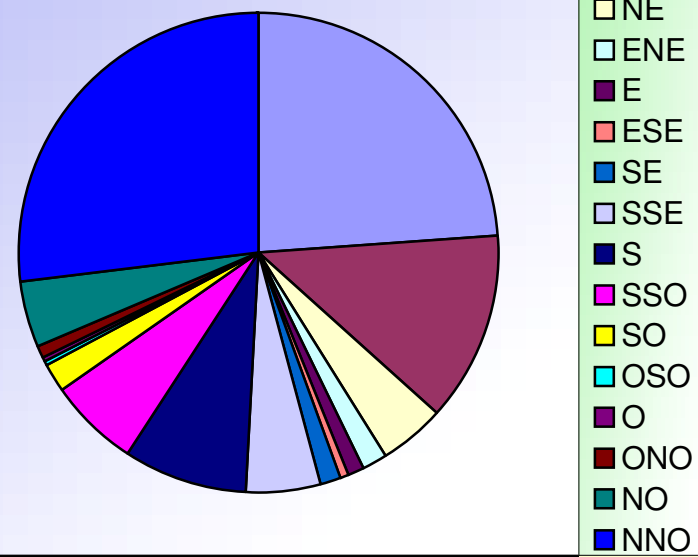
ORIENTATIONS DES VENTS JANVIER 2021
