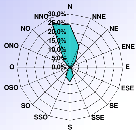
DISTRIBUTION ORIENTATION DU VENT JANVIER 2021
