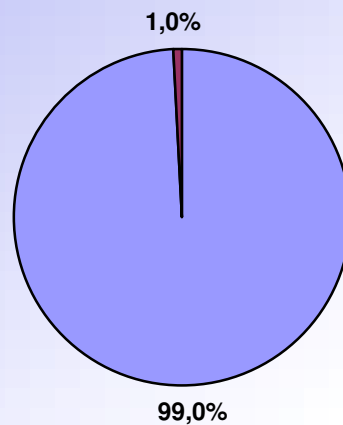
RAPPORT VENT NUL - VENT >0 JANVIER 2021
