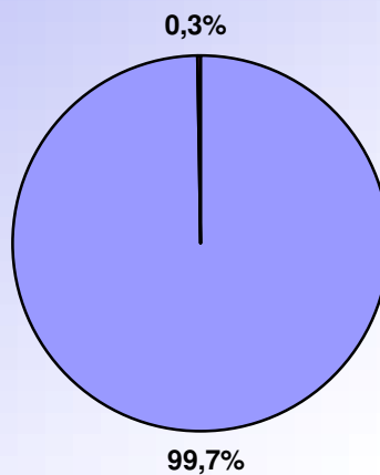
RAPPORT VENT NUL - VENT >0 MAI 2021
