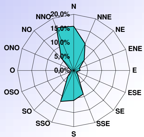
DISTRIBUTION ORIENTATION DU VENT MAI 2021
