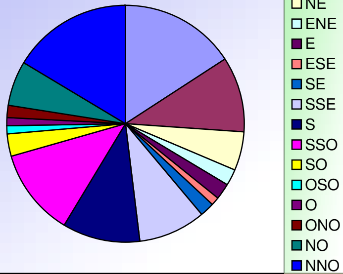
ORIENTATIONS DES VENTS MAI 2021
