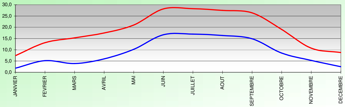
TEMPERATURE (°C) 2021
