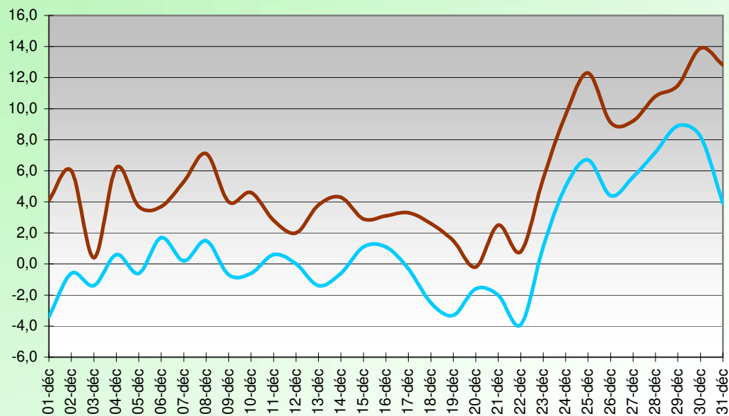
WINDCHILL OU TEMPERATURE RESSENTIE (°C) DECEMBRE 2021
