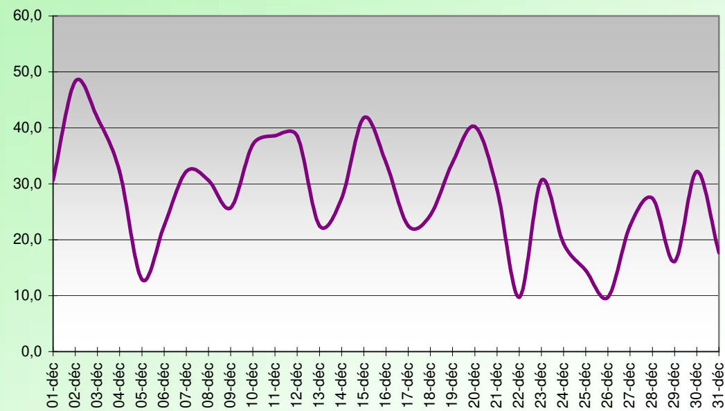
HEAT INDEX OU INDICE DE CHALEUR (°C) DECEMBRE 2021
