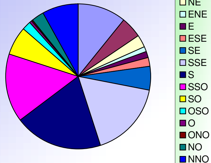
ORIENTATIONS DES VENTS MARS 2022
