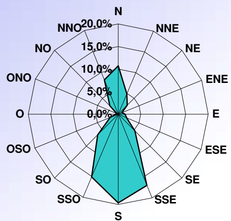
DISTRIBUTION ORIENTATION DU VENT MARS 2022
