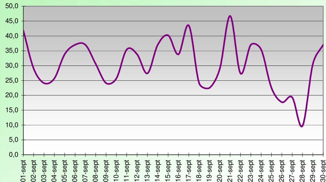
HEAT INDEX OU INDICE DE CHALEUR (°C) SEPTEMBRE 2023
