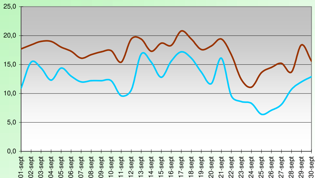
WINDCHILL OU TEMPERATURE RESSENTIE (°C) SEPTEMBRE 2023
