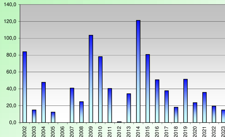
PRECIPITATIONS (mm) FEVRIER
