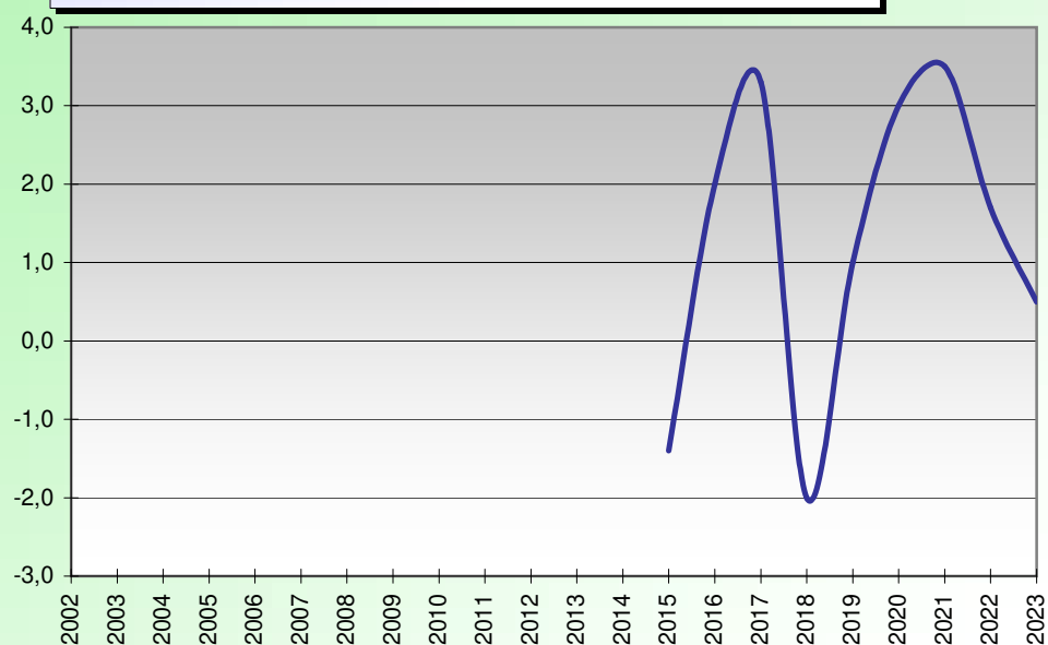
WINDCHILL OU TEMPERATURE RESSENTIE (°C) FEVRIER
