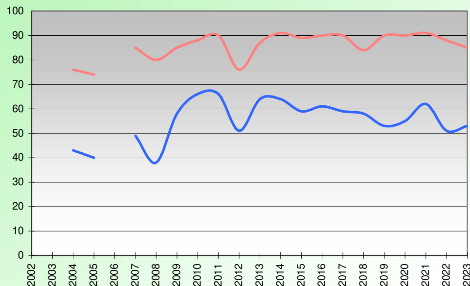
HUMIDITE RELATIVE (%) FEVRIER
