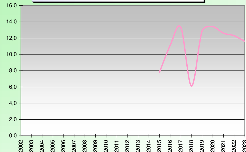
HEAT INDEX OU INDICE DE CHALEUR (°C) FEVRIER
